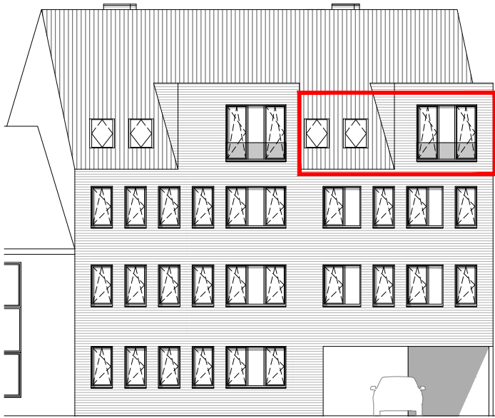
voorgevel - noordwest
